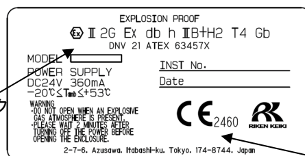
ATEX CE マーキング仕様の銘板例 (DC 電源仕様のみ)
